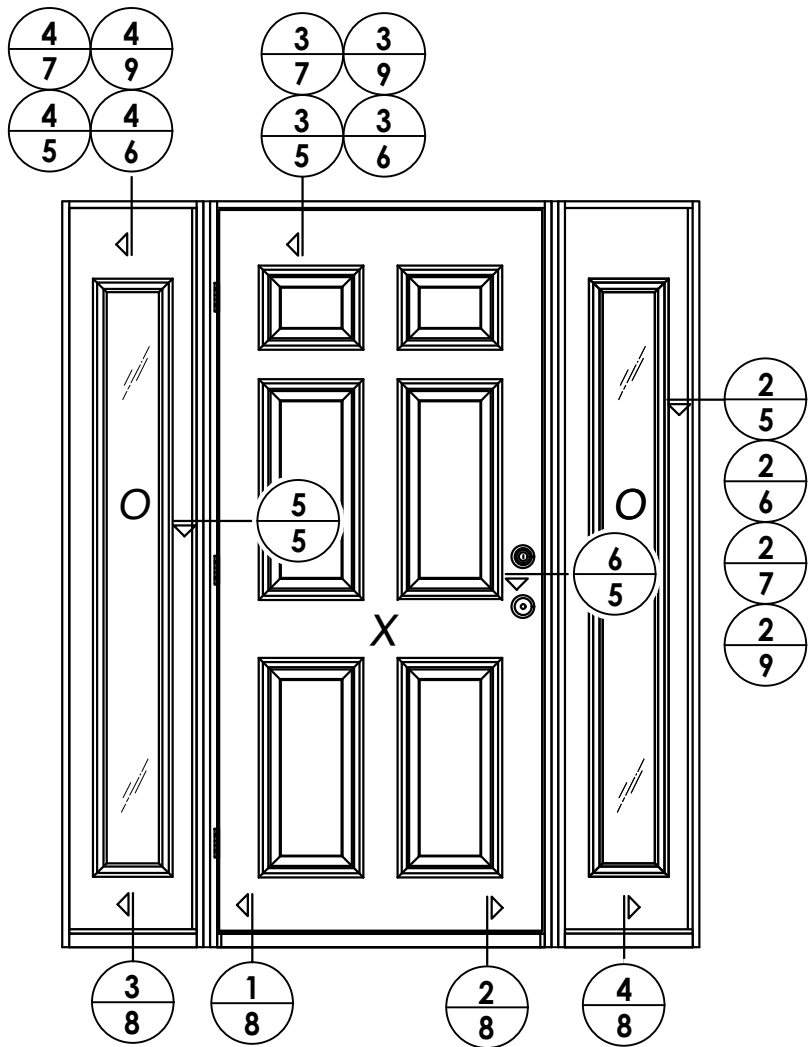
ELEVATION (OXO)
